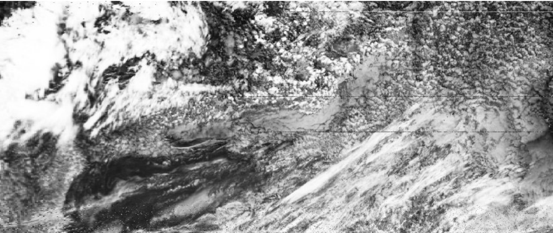
Снимок со спутника METEOR-M2 2, принят на МОПС в Москве. Дата съёмки 06.09.2022 г., 11:23 МСК
